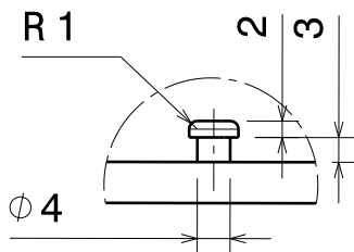
Détail B Echelle : 1:1
